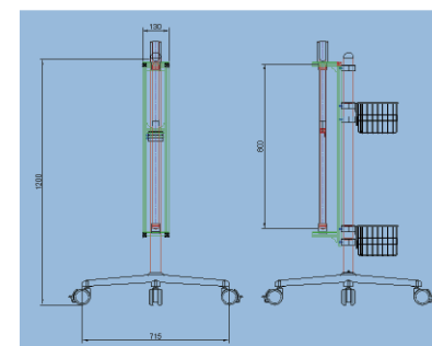
소독관스탠드 카트(1구) KS-RS-SHB1
